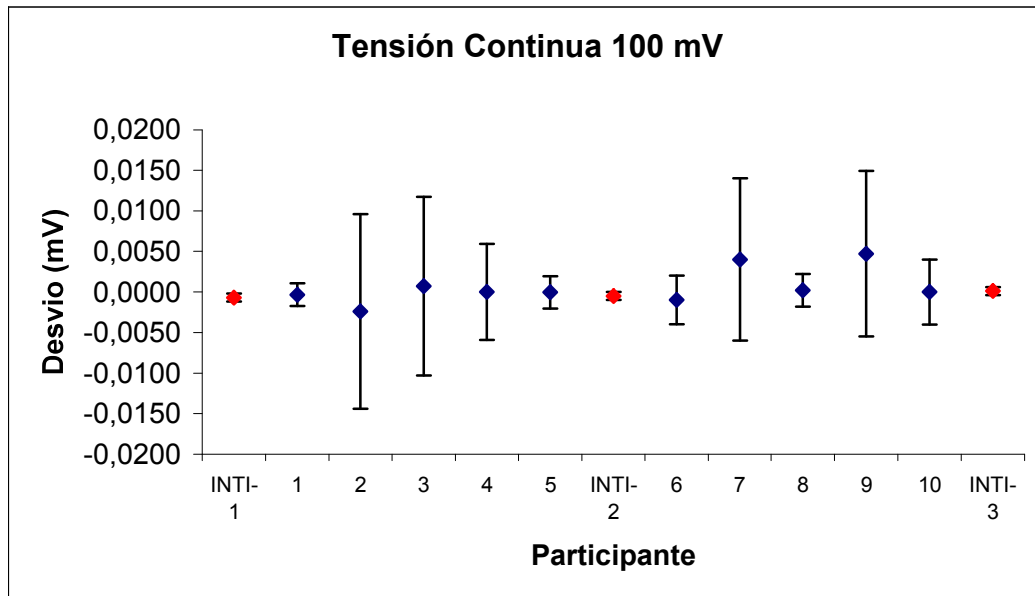
Gráfico 1: Desvíos en tensión continua 100 mV
