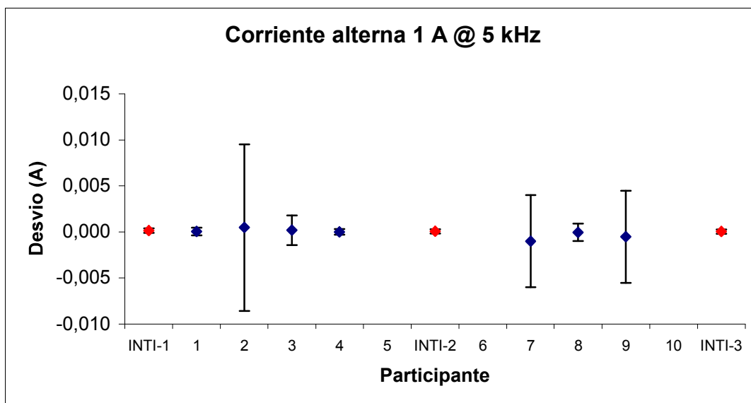
Grafico 12: Desvíos en corriente alterna 1 A @ 5 kHz
