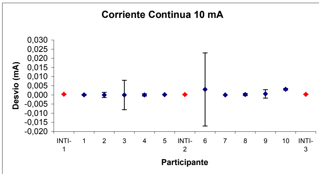
Grafico 4: Desvíos en corriente continua 10 mA
