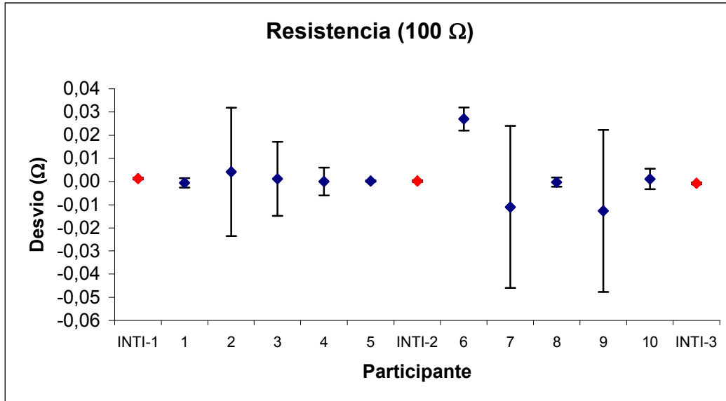
Grafico 13: Desvíos en resistencia 100 Ω
