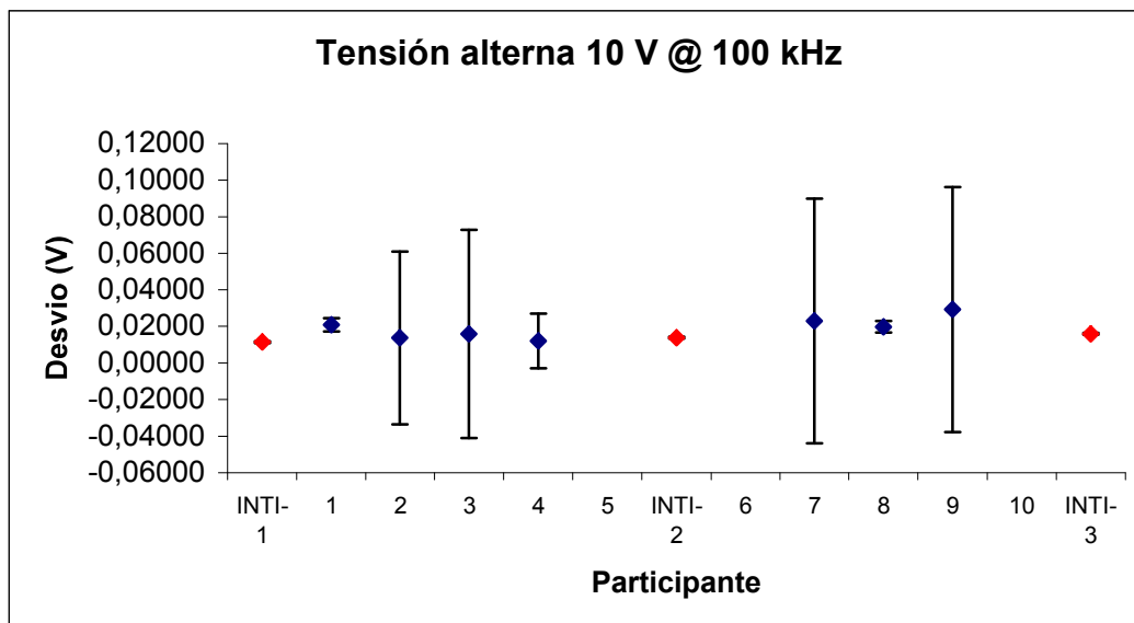
Gráfico 10: Desvíos en tensión alterna 10 V @ 100 kHz
