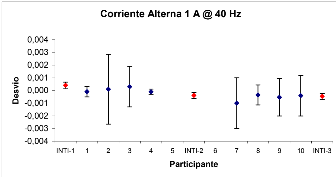
Grafico 11: Desvíos en corriente alterna 1 A @ 40 Hz
