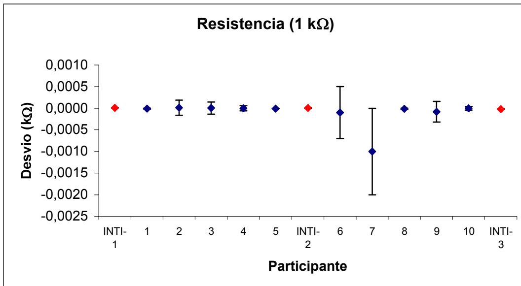
Grafico 14: Desvíos en resistencia 1 kΩ
