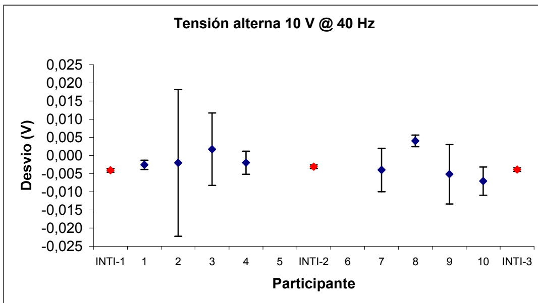
Grafico 8: Desvíos en tensión alterna 10 V @ 40 Hz
