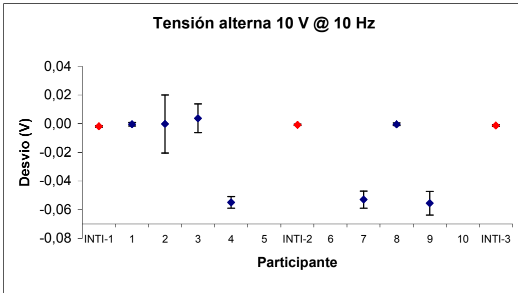
Grafico 7: Desvíos en tensión alterna 10 V @ 10 Hz
