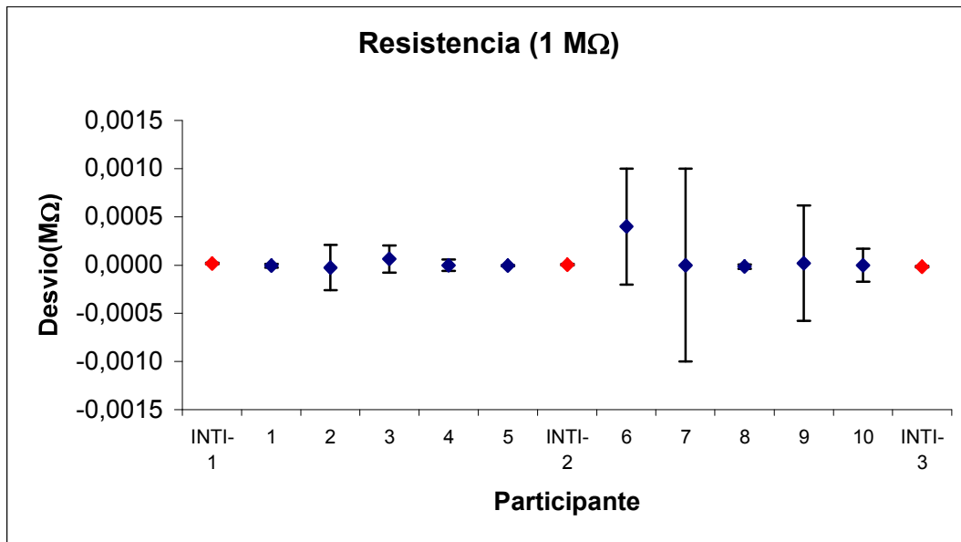
Grafico 15: Desvíos en resistencia 1 MΩ
