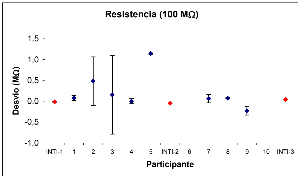
Grafico 16: Desvíos en resistencia 100 MΩ
