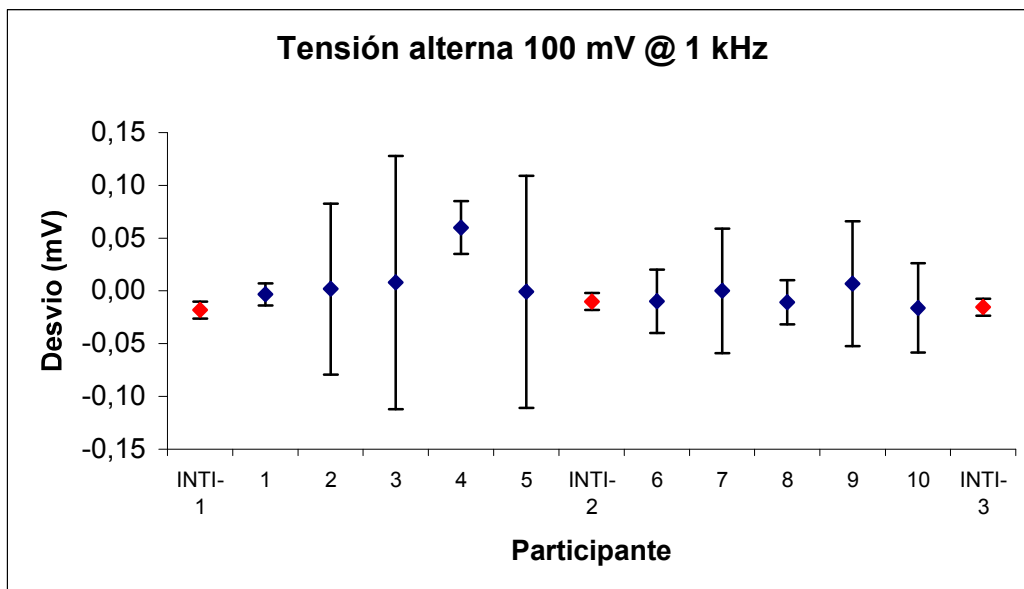
Grafico 6: Desvíos en tensión alterna 100 mV @ 1 kHz
