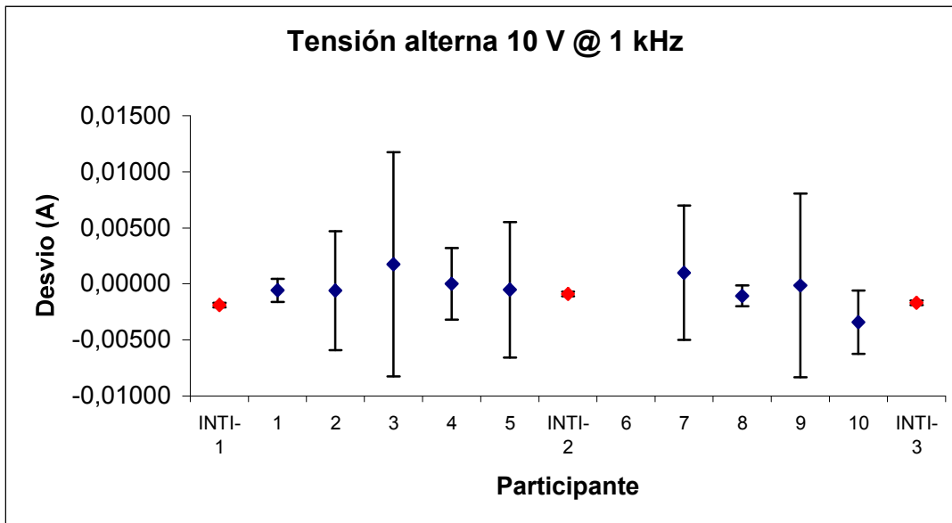
Gráfico 9: Desvíos en tensión alterna 10 V @ 1 kHz
