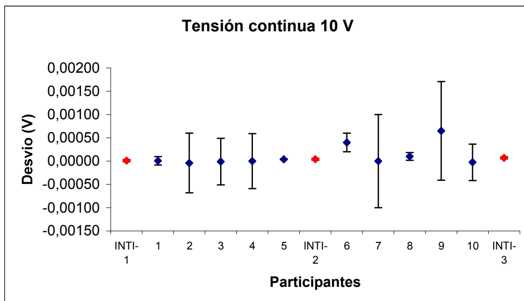
Gráfico 2: Desvíos en tensión continua 10 V
