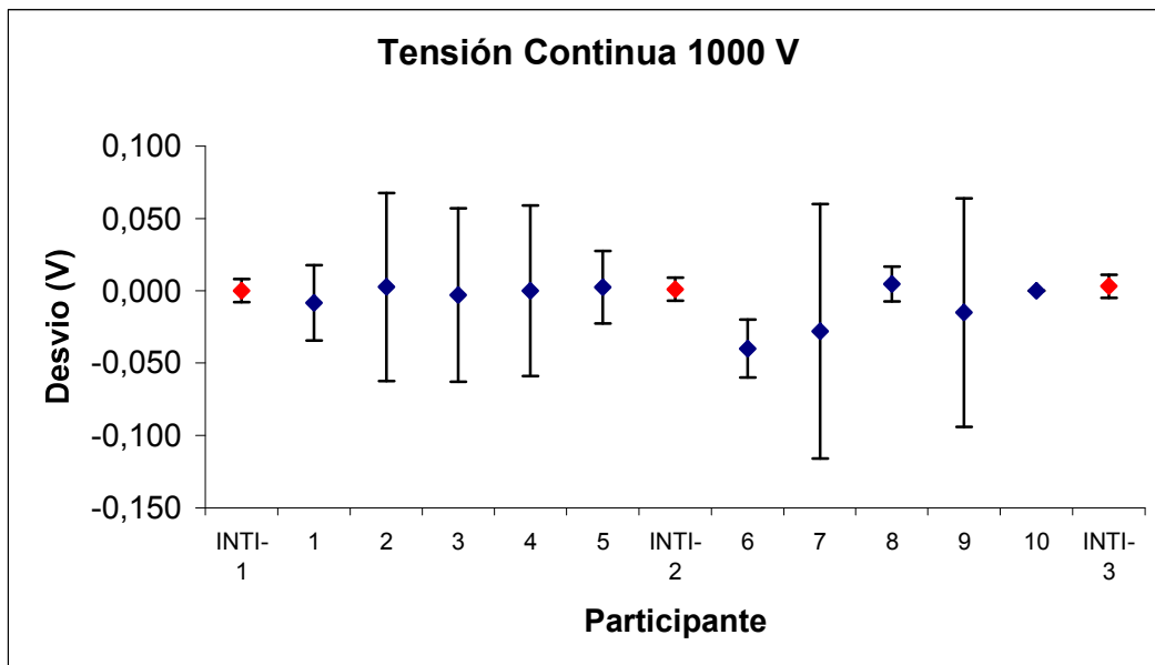
Grafico 3: Desvíos en tensión continua 1000 V
