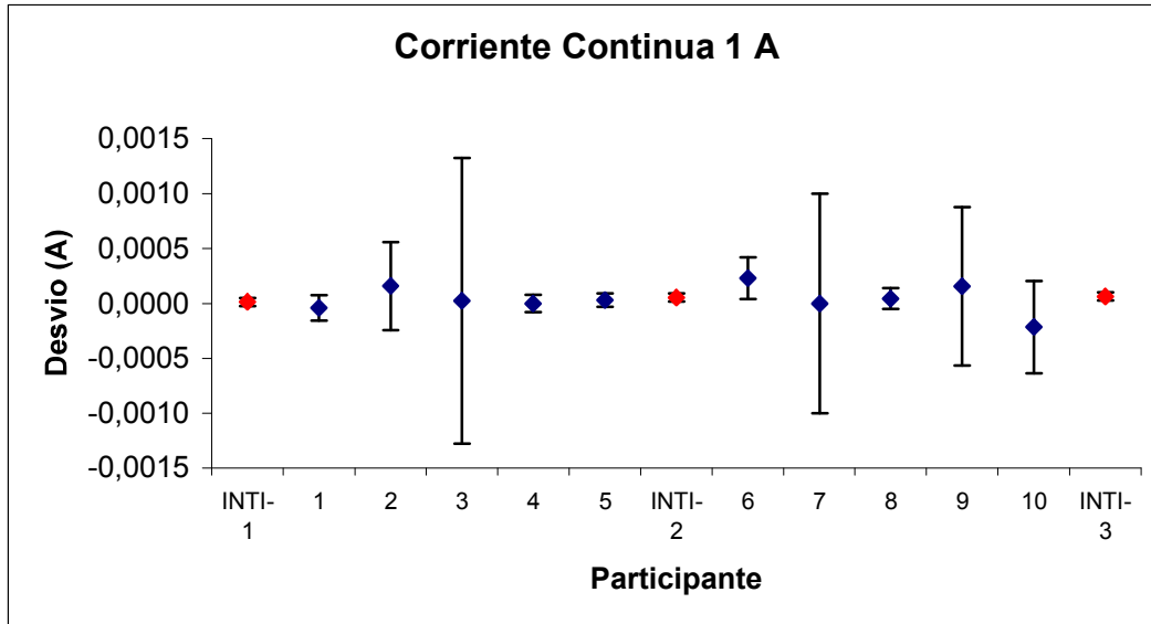
Grafico 5: Desvíos en corriente continua 1 A
